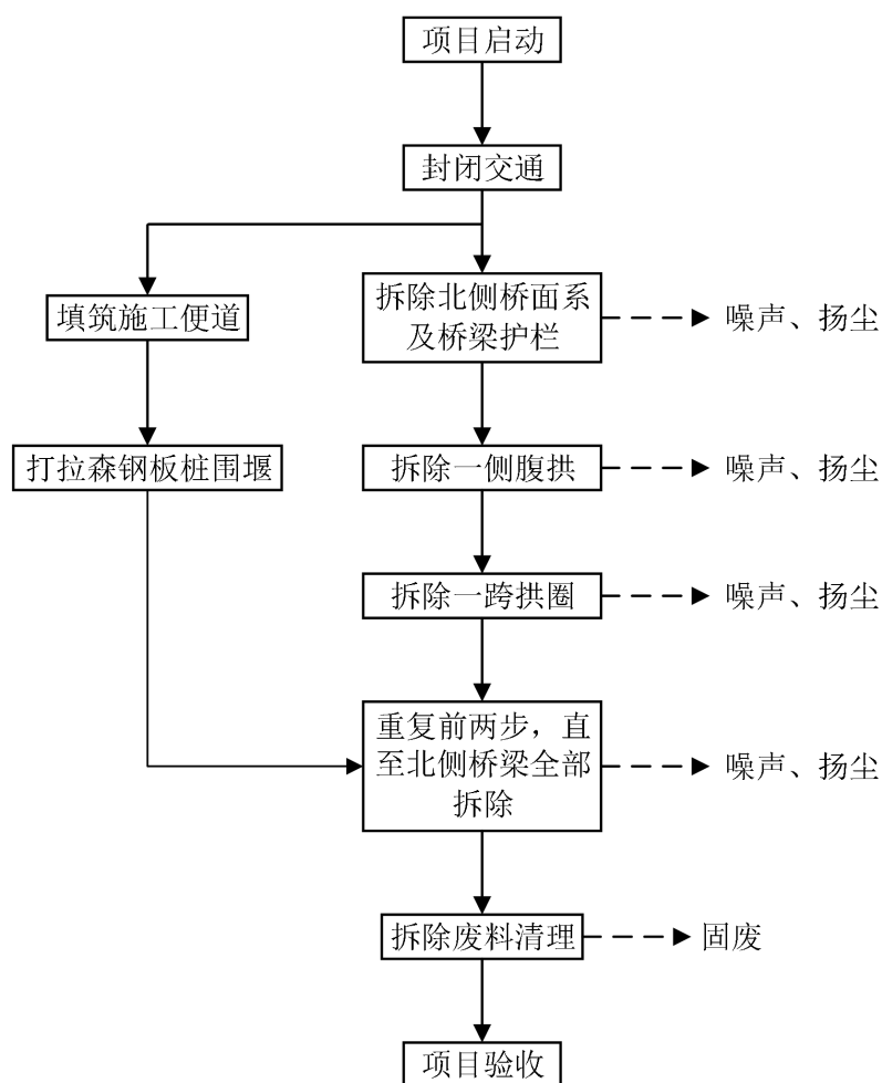
图 2-1 旧桥拆除施工工艺流程及产污环节图
